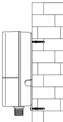
Установка патрубками вниз
