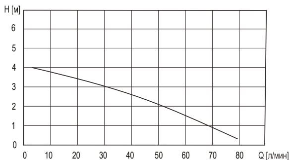
Рис. 1. Гидравлические характеристики.
