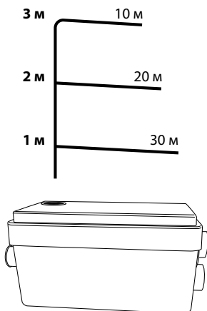
Рис. 4. Максимальная длина трубопровода.
