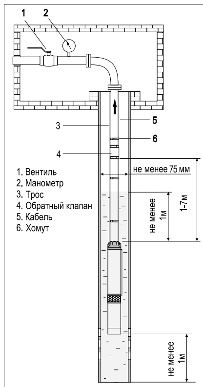
Рис. 2. Монтаж насоса.
